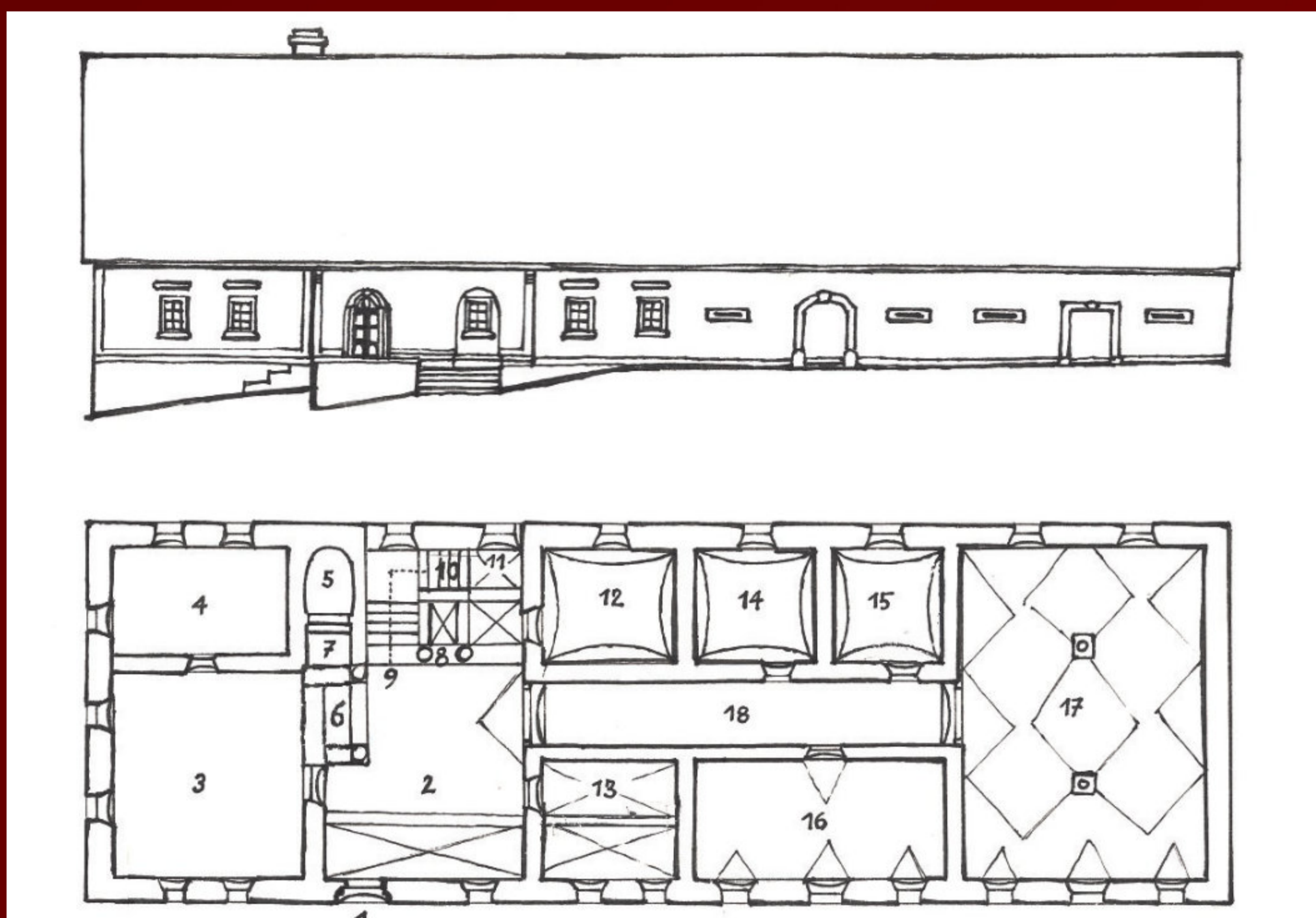
PŘÍKLAD SCHÉMATU STATKU BROUMOVSKÉHO TYPU
